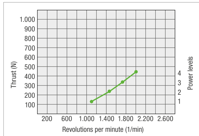
SEABOB F5
